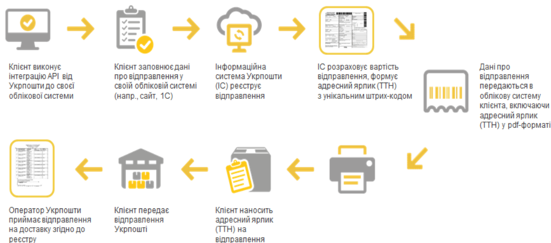
Рис. 1.1. Схематичне зображення процесу роботи з API
